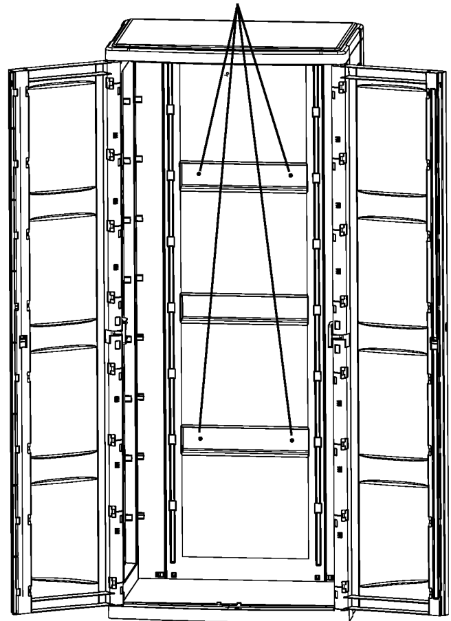
Cabinet Mounting Holes / Emplacement des trous de montage de l'armoire. / Perforaciones de Montaje en el Gabinete
